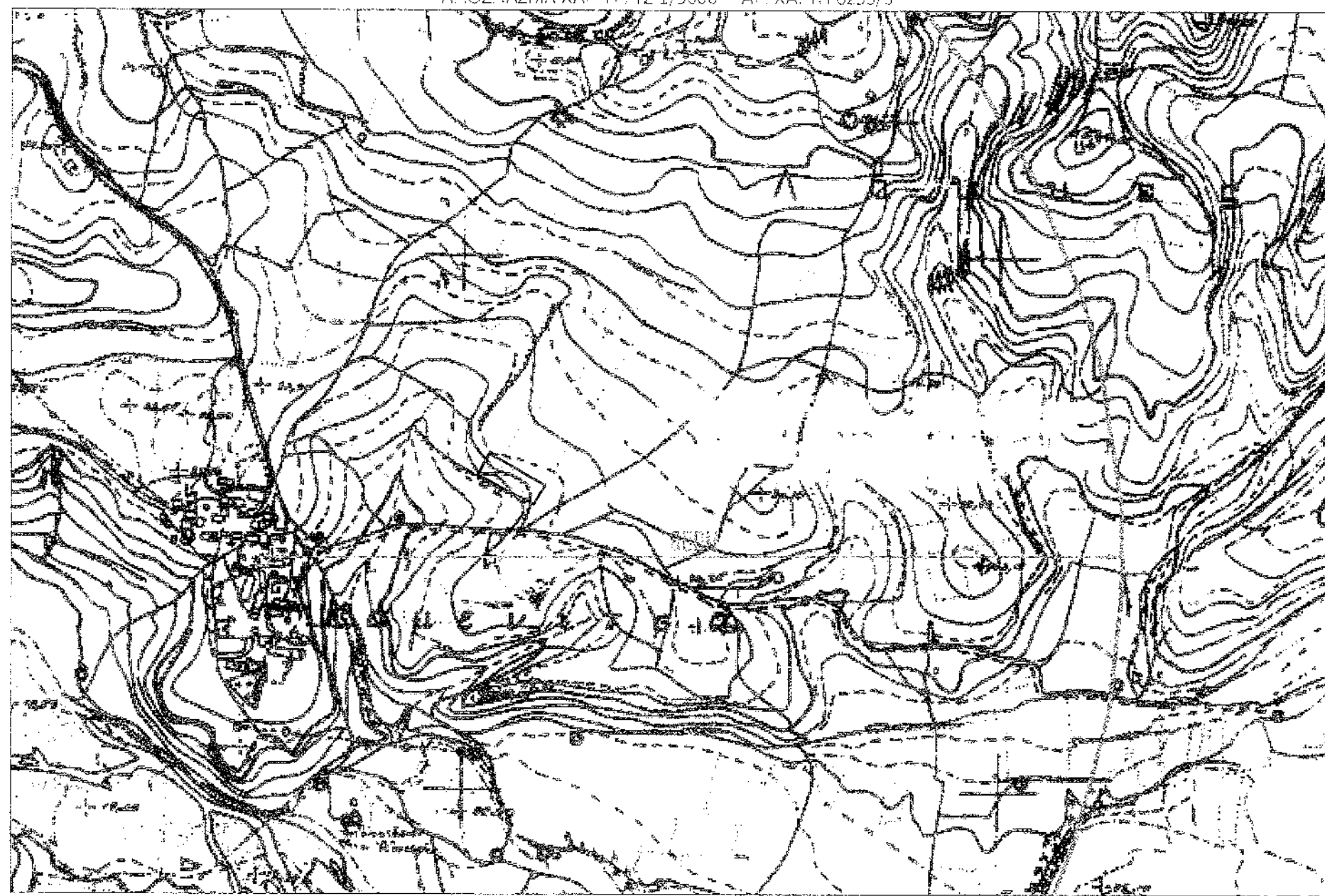
ΟΔΟΓΡΑΦΙΚΟ ΣΚΑΡΙΦΗΜΑ
