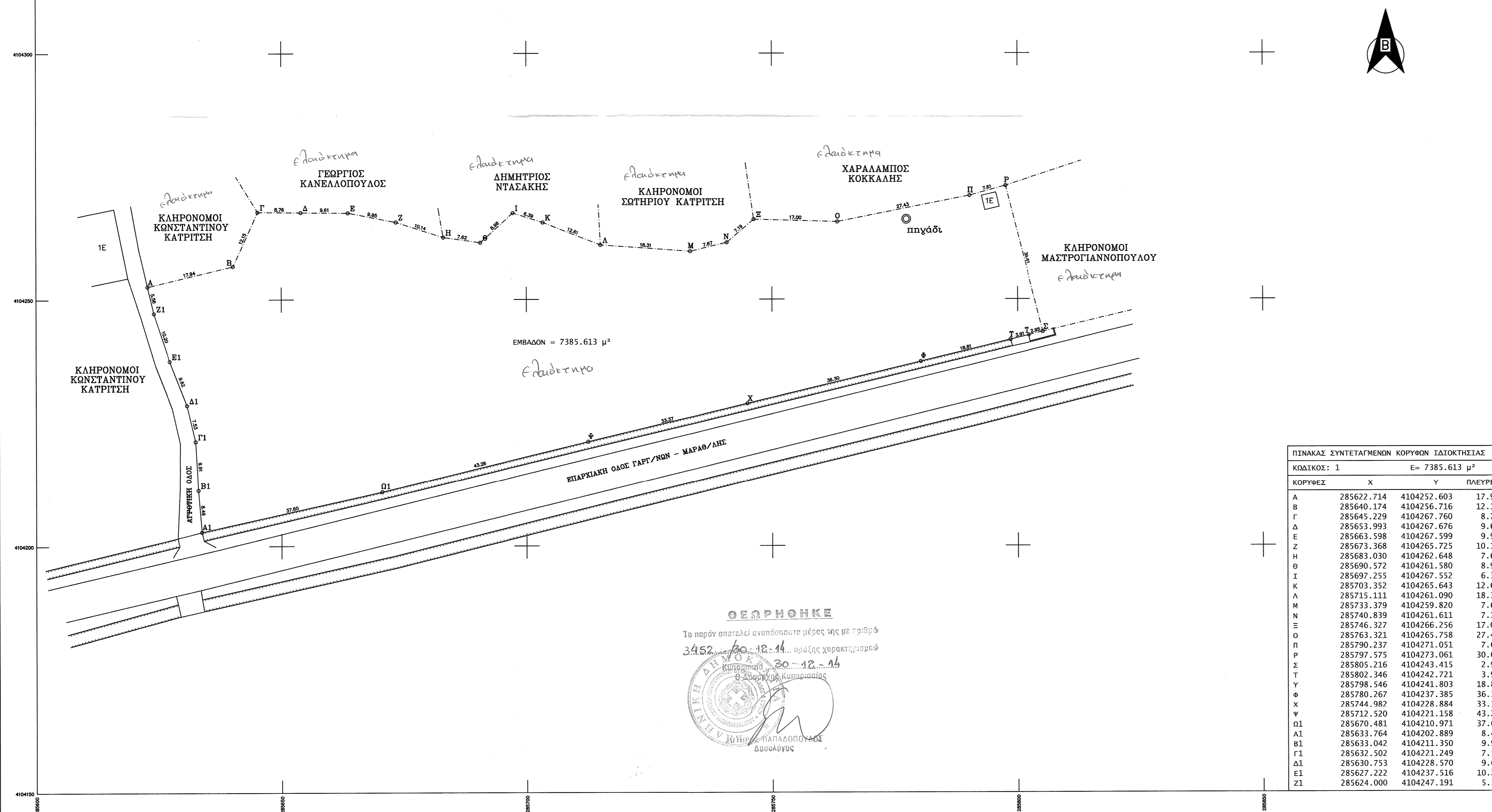
ΑΠΟΣΠΑΣΜΑ ΑΠΟ ΦΧ ΤΗΣ ΓΥΣ ΚΛΙΜΑΚΑ 1:5000 7243/4
