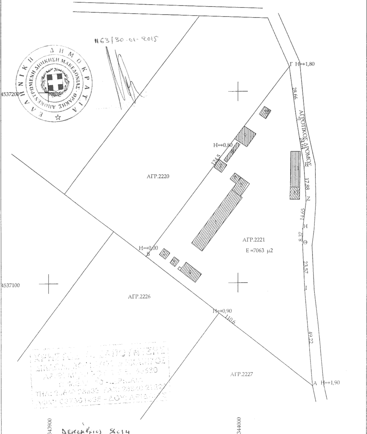
Τοπογραφικό Διάγραμμα
