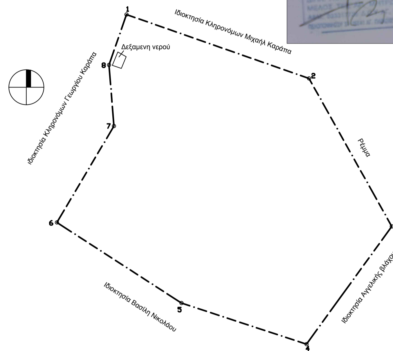
ΤΟΠΟΓΡΑΦΙΚΟ ΔΙΑΓΡΑΜΜΑ ΚΛ. 1:500
