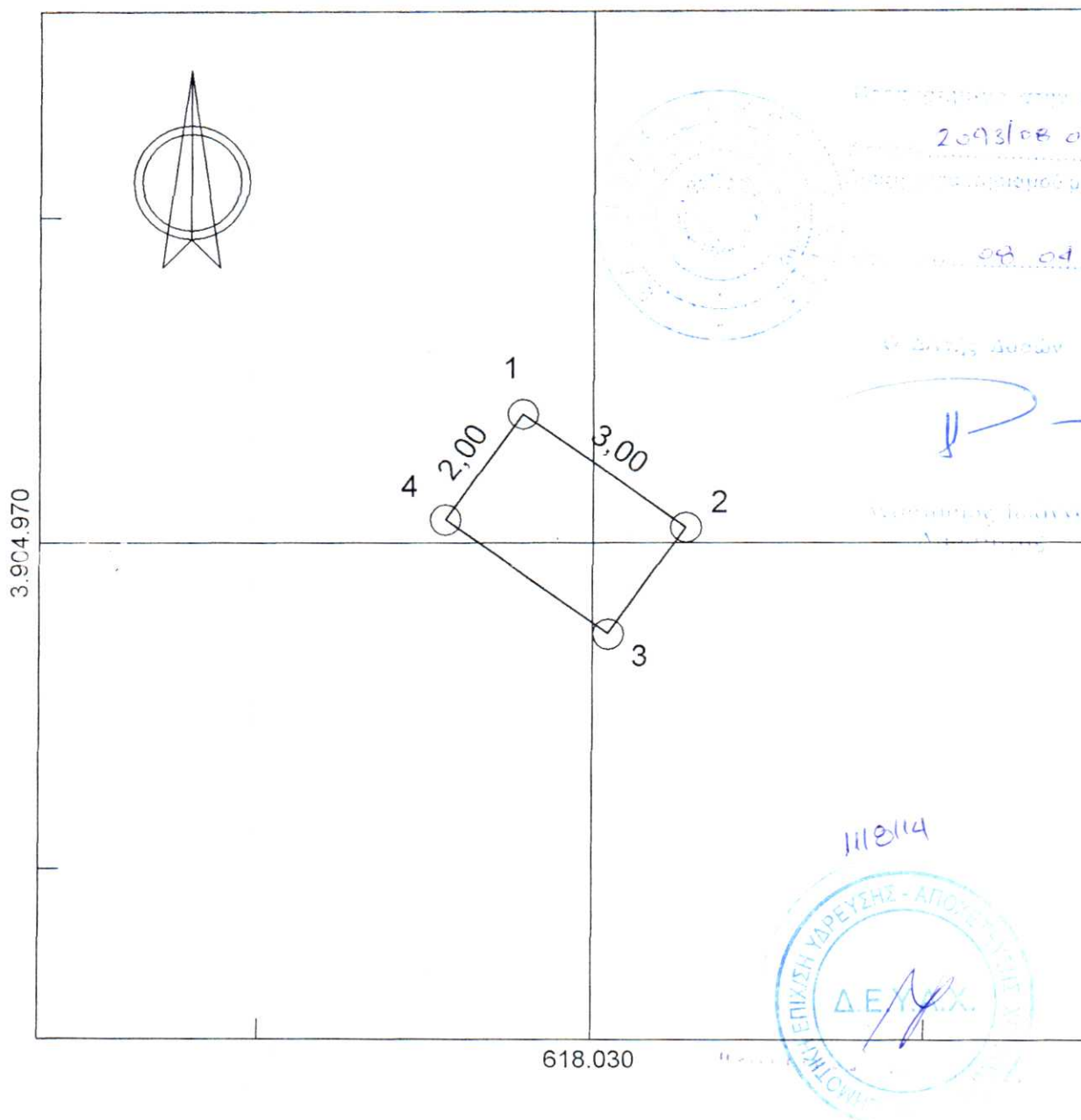
Πίνακας Συντεταγμένων των κορυφών του 1,2,3,4,1 Εμβαδόν τεμαχίου = 6,00 τ.μ. - Περίμετρος = 10,00 μ.
