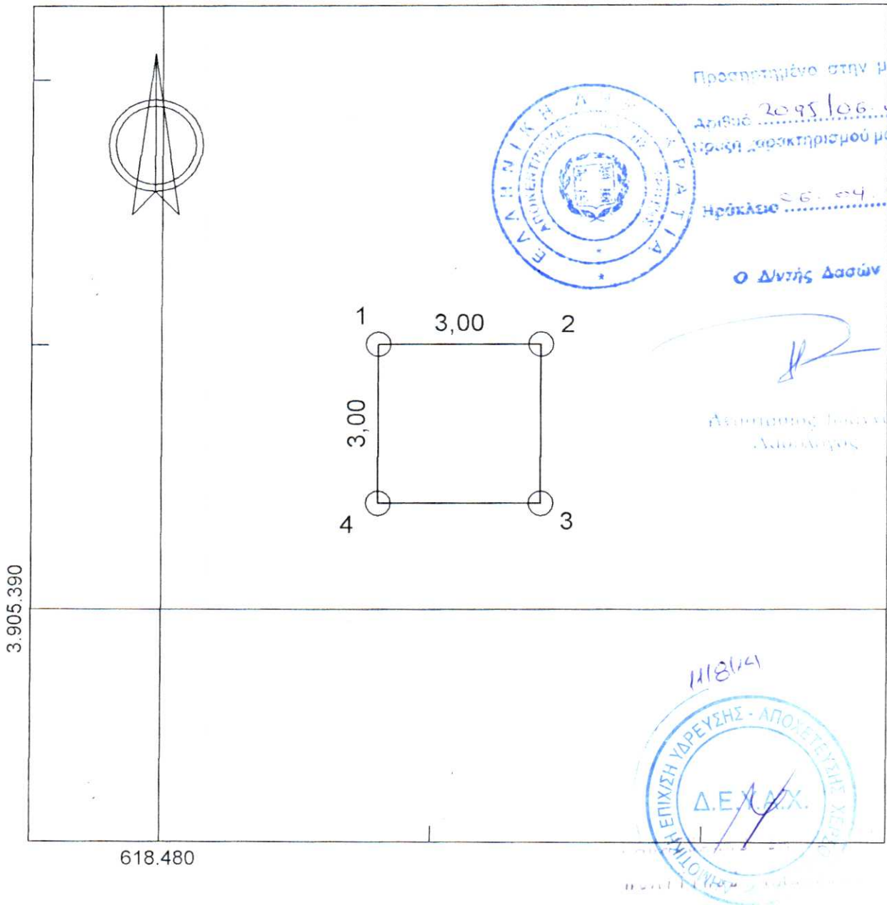
Πίνακας Συντεταγμένων των κορυφών του 1,2,3,4,1 Εμβαδόν τεμαχίου = 9,00 τ.μ. - Περίμετρος = 12,00 μ.
