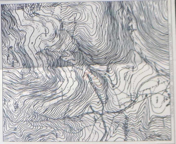
ΑΝΟΡΘΩΤΟ ΟΡΟΓΡΑΦΙΚΟ ΧΑΡΤΟΧΕΙΡΩΝ ΣΤΕΡΕΟΣΧΗΜΑΤΟΣ 2017-2020
