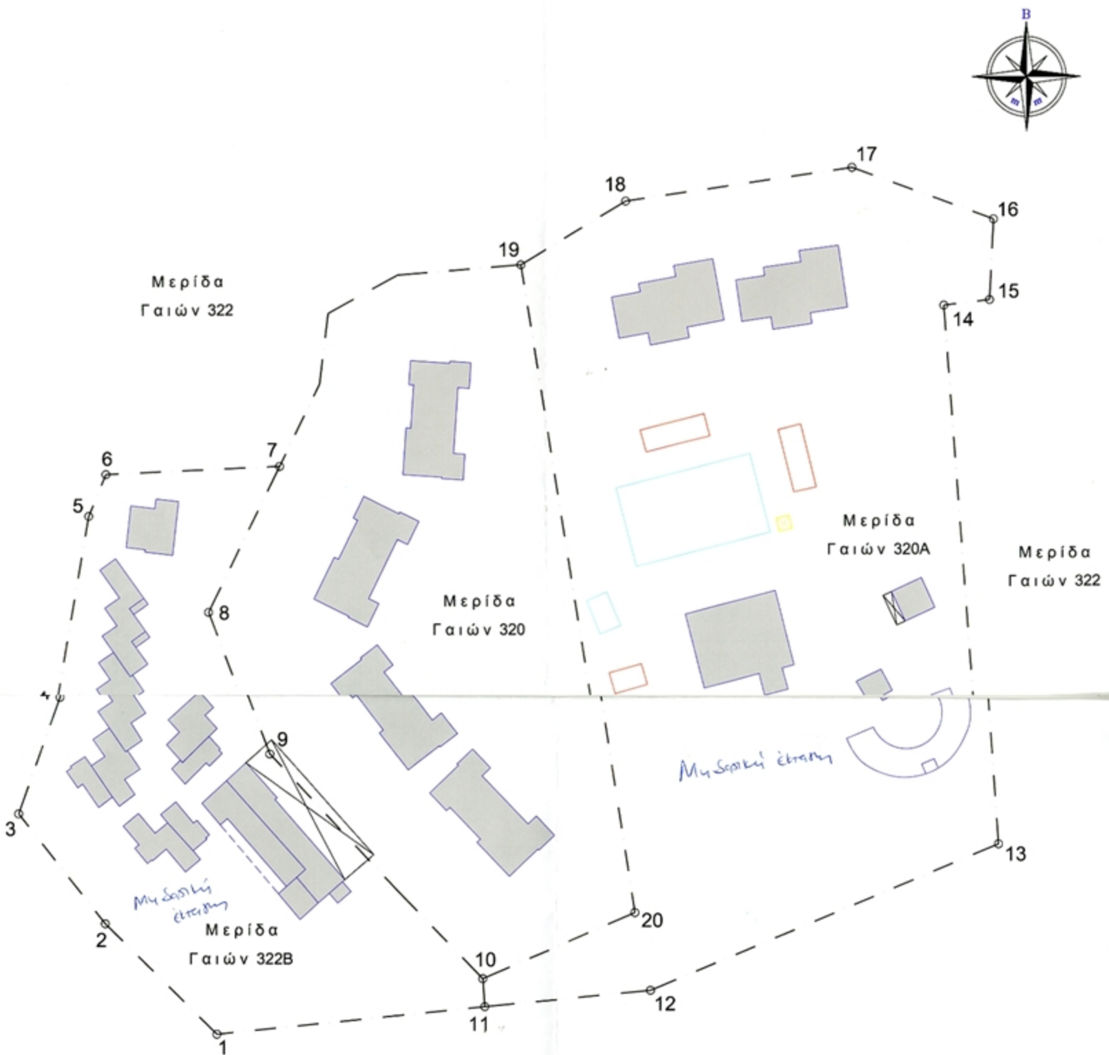
ΣΥΝΤΕΤΑΓΜΕΝΕΣ ΚΟΡΥΦΩΝ Μ.Γ. 322Β
