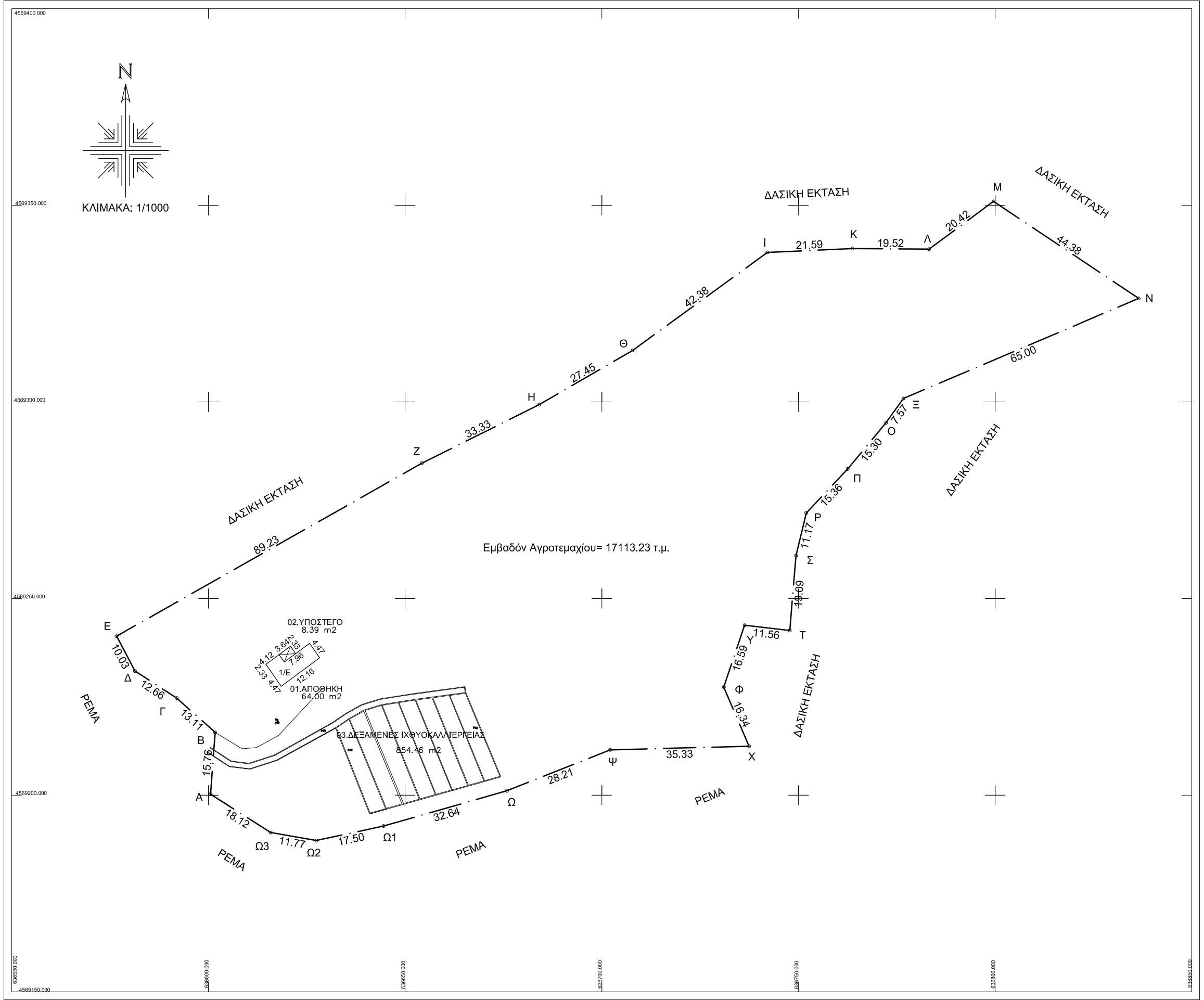
ΤΟΠΟΓΡΑΦΙΚΟ ΔΙΑΓΡΑΜΜΑ ΑΓΡΟΤΕΜΑΧΙΟΥ
