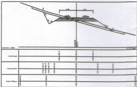
ΤΥΠΙΚΗ ΔΙΑΤΟΜΗ
