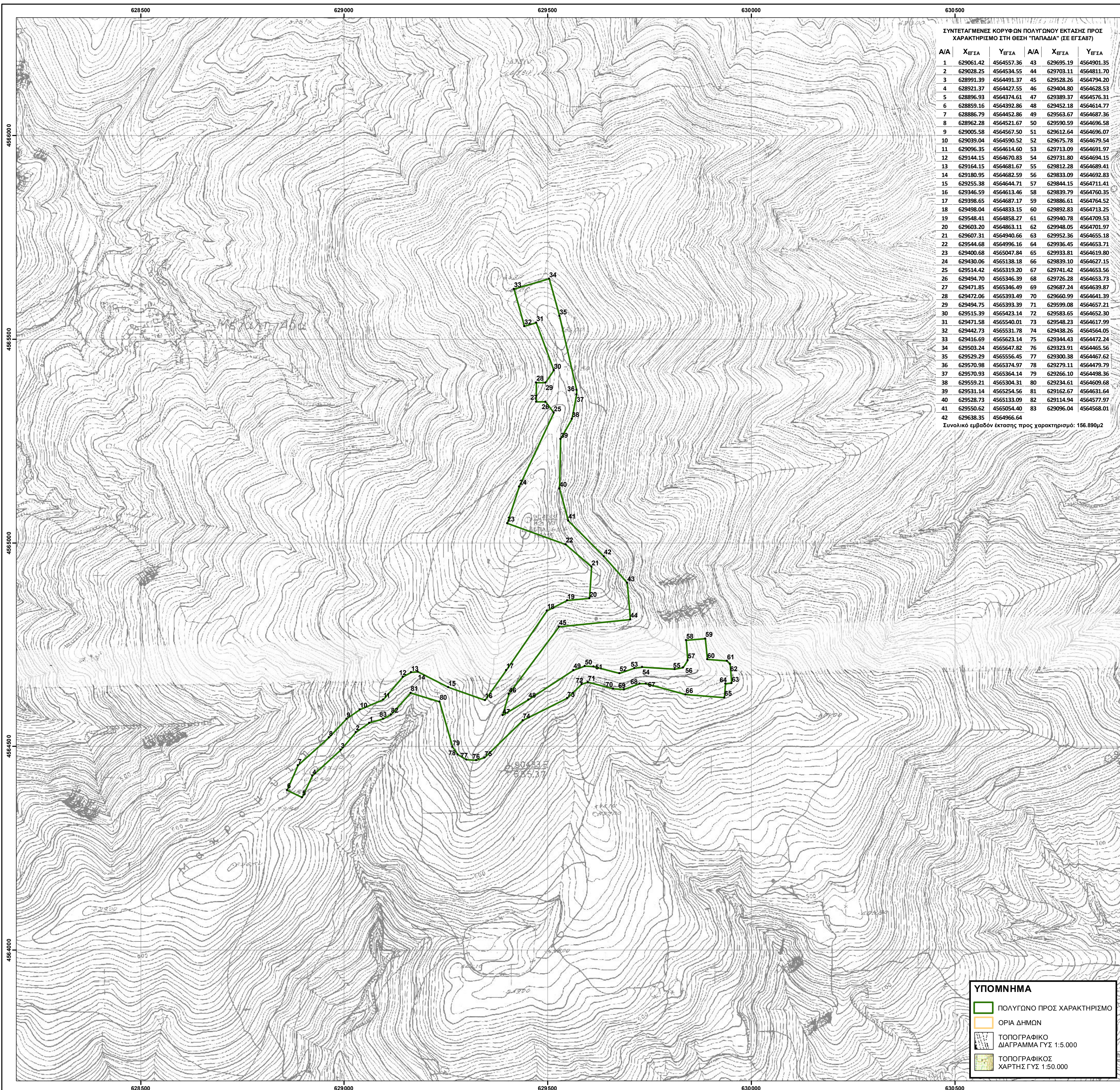
Τοπογραφικό Διαγράμμα Γ.Υ.Σ. 1:5.000
