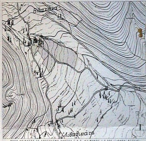
ΒΕΛΛΑ ΚΙΝΗΤΟΥ ΣΣ ΑΡΧΙΤΕΚΤΟΝΙΚΟ ΣΧΗΜΑ ΣΧΗΤΟΥ Γ. Σ. ΚΑΙΜΑΚΟΣ 1:8.000 (ΓΙΔΑΡΗ 612314)
