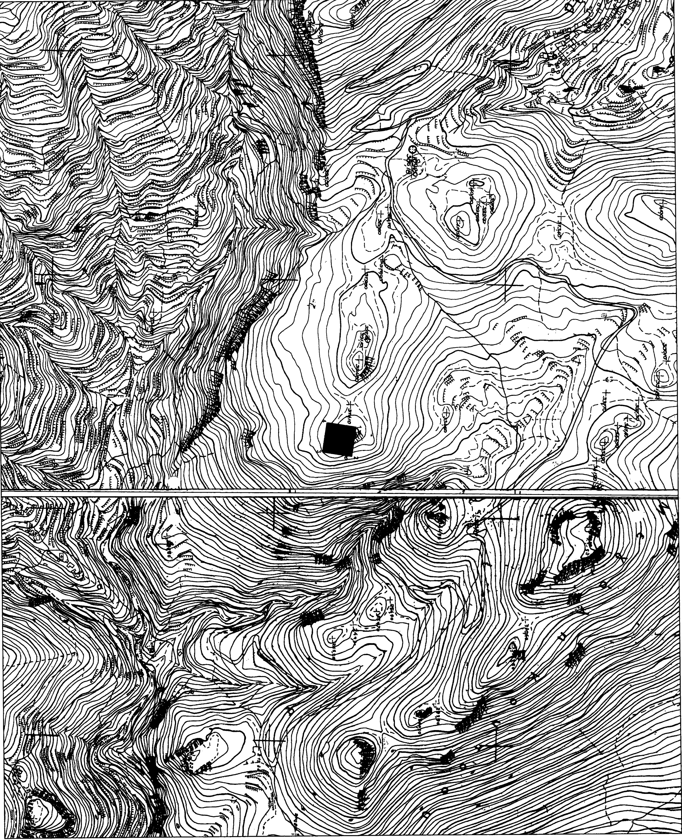
ΑΠΟΤΥΠΩΣΗ ΠΟΛΥΓΩΝΟΥ ΓΗΠΕΔΟΥ ΕΚΚΑΤΑΣΤΑΣΗΣ Α. ΣΕ Κ. ΜΑΚΑΣ 1:5.000 (Φ.Χ. ΓΥΣ 1:5.000 7398/6 & 7399/5)
