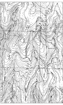
ΑΝΘΙΣΤΑΣΙΑ ΧΑΡΤΗ 1:2.5 (1:5.000) Φύλλο Μαγνήσι 4243 Απόκλιση από Ν.Α. Υψόμετρο 116,000
