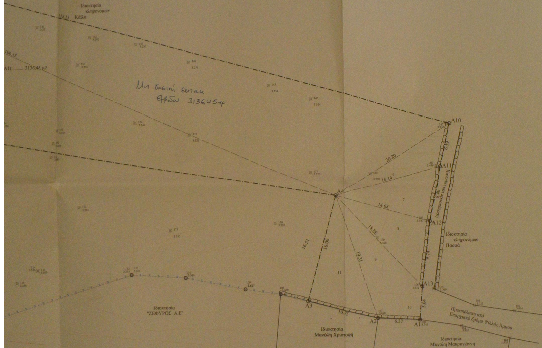
ΤΟΠΟΓΡΑΦΙΚΟ ΔΙΑΓΡΑΜΜΑ κλίμακα 1:200
