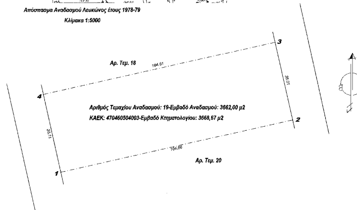
Τοπογραφικό Διάγραμμα κλ. 1:500
