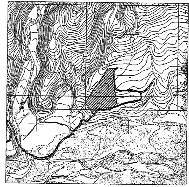
ΑΠΟΣΠΑΣΜΑ ΔΙΑΓΡΑΜΜΑΤΟΣ 1:5000 Γ.Υ.Σ. 7205-7+7215-1
