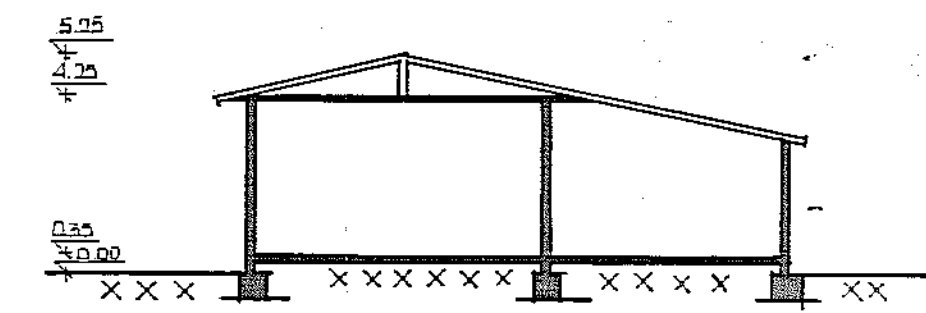
Σημειωμένη τομή
