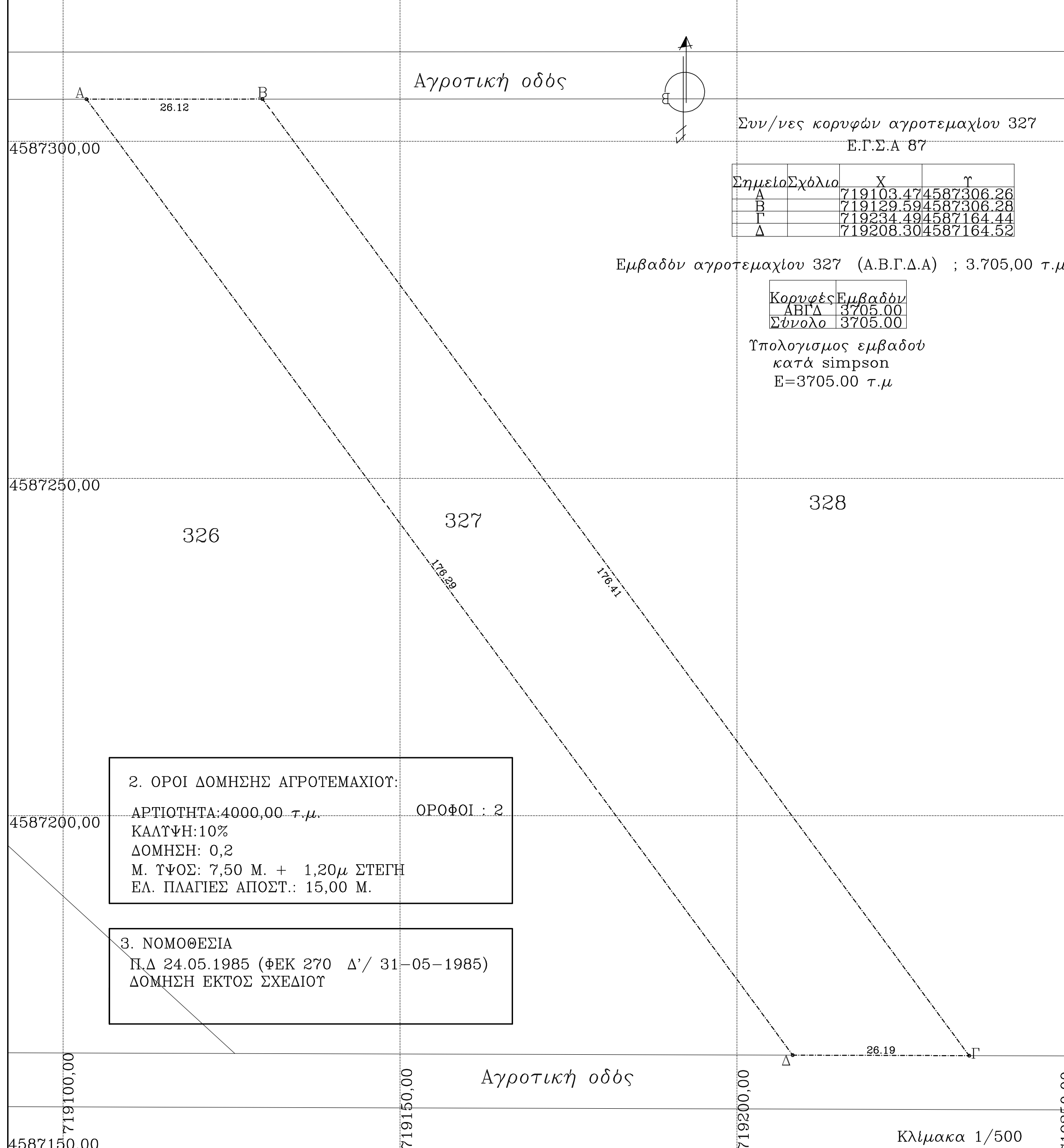
Τοπογραφικό διάγραμμα
