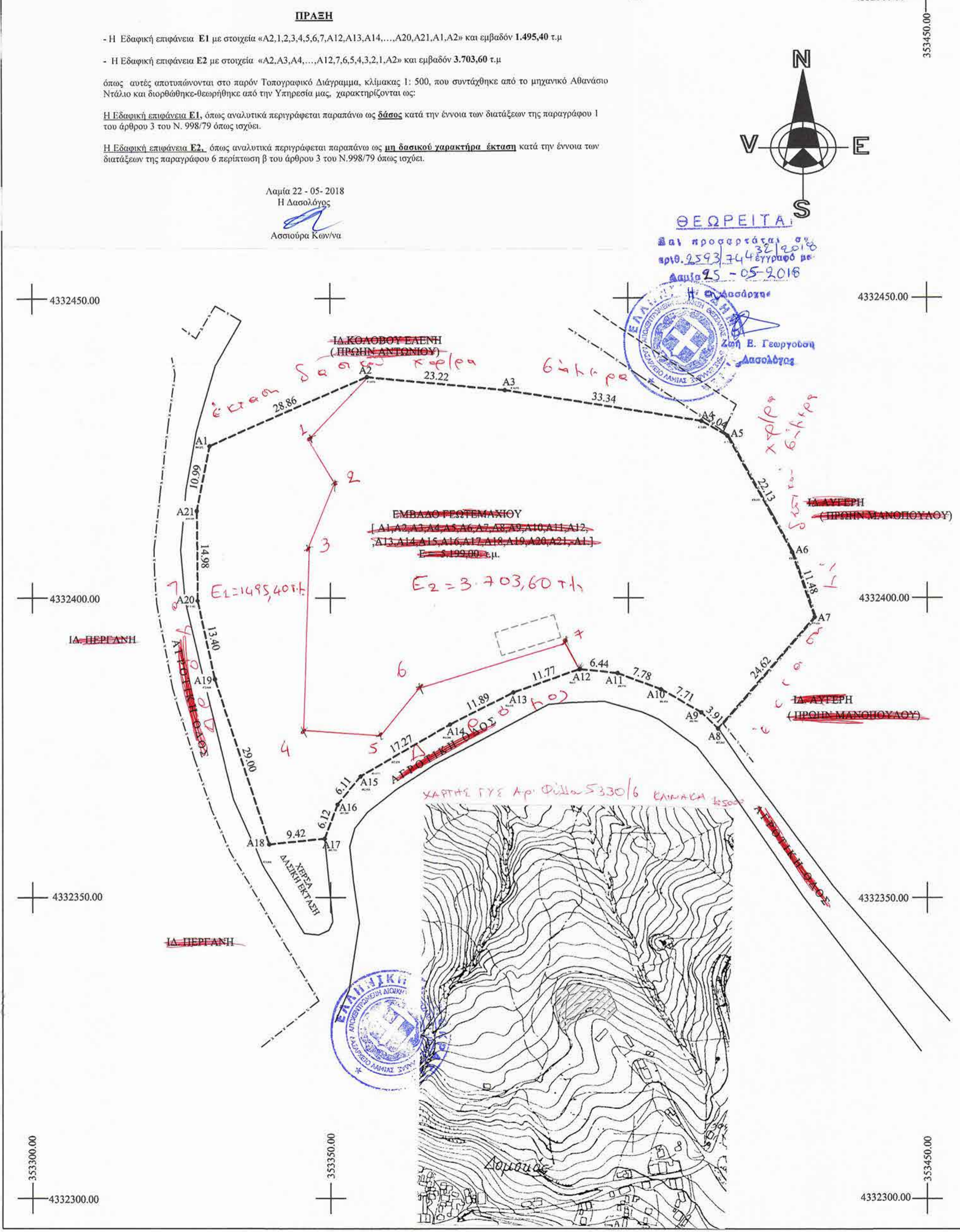
ΣΥΝΤΕΤΑΓΜΕΝΕΣ ΚΟΡΥΦΕΣ-ΣΗΜΕΙΩΝ ΑΓΡΟΤΕΜΑΧΙΟΥ ΕΓΣΑ 87 ΕΓΚΑΡΣΙΑ ΜΕΡΚΑΤΟΡΙΚΗ, ΠΡΟΒΟΛΗ U.T.M. ΕΛΛΗΝΙΣΤΡΩΦΕΙΣ GRS 80, Φ.Χ. 1:50.000
