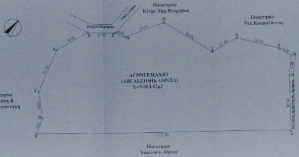
ΤΟΠΟΓΡΑΦΙΚΟ ΔΙΑΓΡΑΜΜΑ ΚΛΙΜΑΚΑ 1:500
