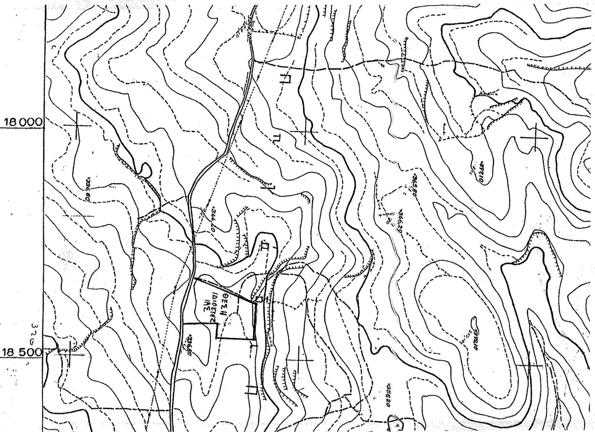
ΑΠΟΣΤΑΣΜΑ ΧΑΡΤΗ Γ.Υ.Σ. ΑΡ. ΦΥΛΛΟΥ 5399/2 ΚΑΙ 1:5000
